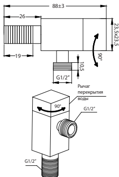
Угловой вентиль G1/2" на G3/4"
