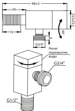
Угловой вентиль G1/2" на G1/2"
