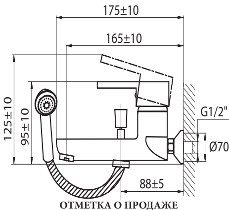
Схема для смесителя Krona
