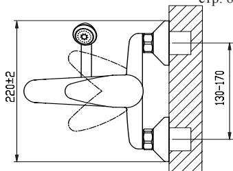
Схема для смесителя Krona
