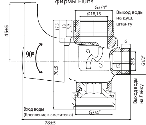
Схема №2 (Вариант №2) Рабочий элемент фирмы Fluhs
